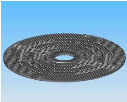
Der Interkonnektor: Dieses CD-grosse, metallische Verbindungsstück trennt jeweils zwei Brennstoffzellen voneinander. Das Oberflächenprofil ermöglicht das Durchströmen des Synthesegases, mit dem die Brennstoffzellen betrieben werden.
