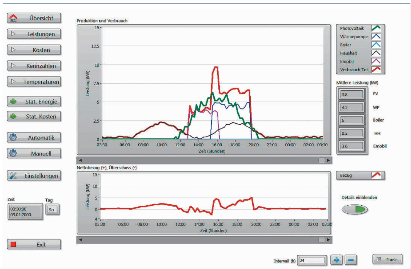
Abb. 8: Bedienoberfläche mit Leistungsverläufen (kW) für alle Produzenten und Verbraucher (oben) und aktueller Leistungsbilanz (unten: positive Werte für Bezug, negative Werte für Einspeisung).
