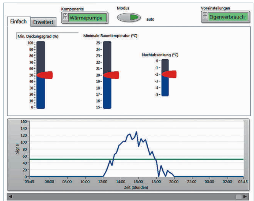
Abb. 9: Automatik-Modus für die Optimierung des Eigenverbrauchs, Beispiel Wärmepumpe. Vorgabewerte sind der minimale solare Deckungsgrad in % (Schiebereglers links) sowie die minimale Raumtemperatur in °C (Schiebereglers Mitte und rechts für Nachtabsenkung). Im Plot unten ist der Verlauf des solaren Deckungsgrads (blau) sowie der vorgegebene Schwellwert (grün) dargestellt. Beim Überschreiten des Schwellwerts wird die Wärmepumpe eingeschaltet.
