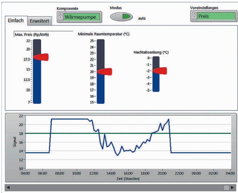
Abb. 10: Automatik-Modus für die Optimierung der Kosten, Beispiel Wärmepumpe. Vorgabewerte sind die Preisgrenze in Rp./kWh (Schieberegler links) sowie die minimale Raumtemperatur in °C (Schieberegler Mitte/rechts). Im Plot unten ist der Verlauf des variablen Strompreises (blau) sowie die vorgegebene Preisgrenze (grün) dargestellt. Beim Unterschreiten der Preisgrenze wird die Wärmepumpe eingeschaltet.
